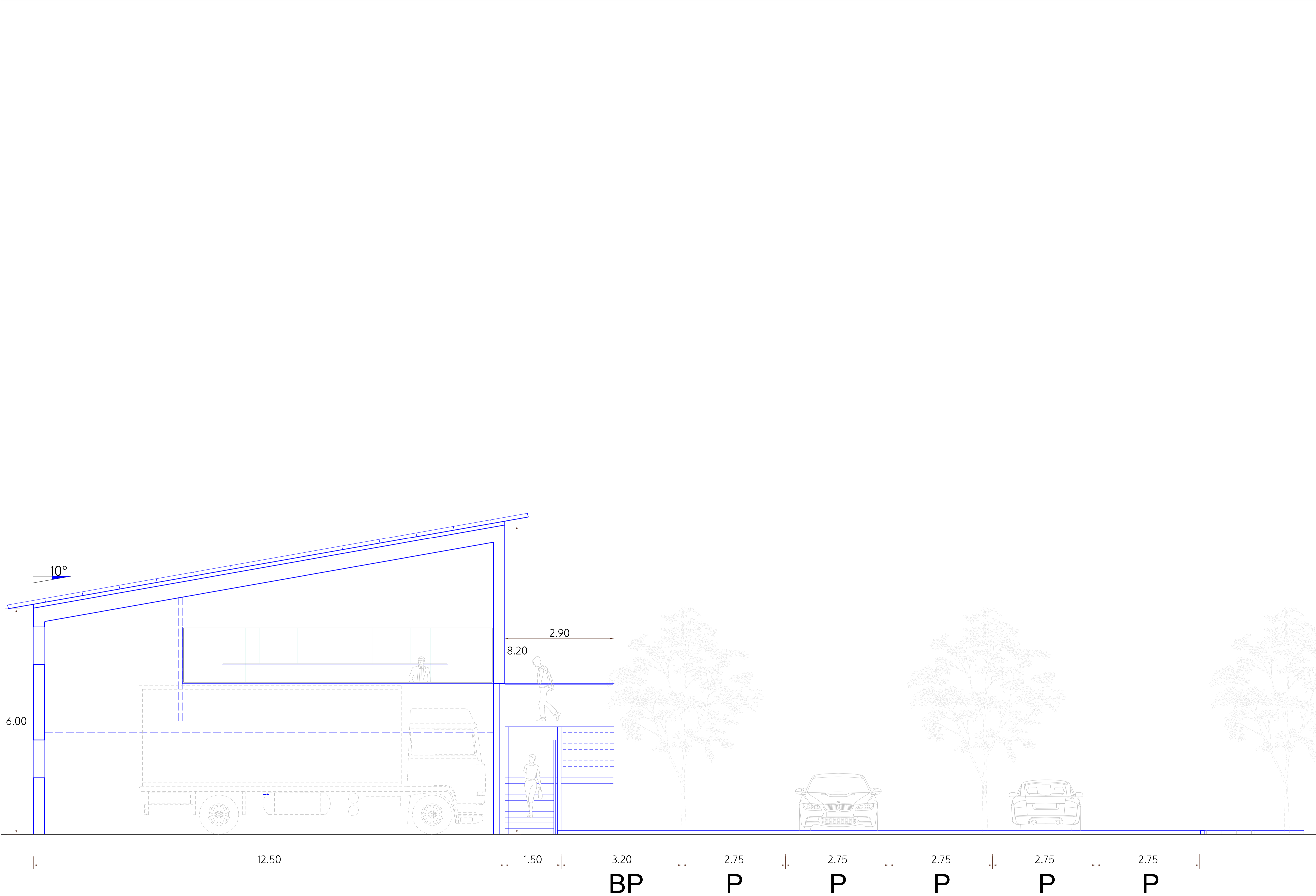
Schnitt A-A
